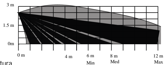
Vista laterale
